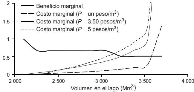
GRÁFICA 1. Beneficio y costo marginal de tener agua en el lago (Pesos/m 3 )
